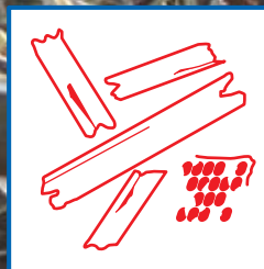
Crop residues
